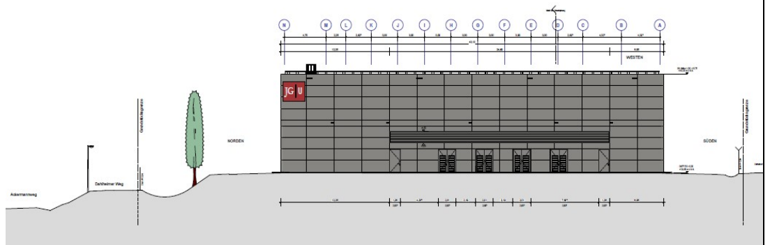
Ansicht Westen, Koblenzer Straße
