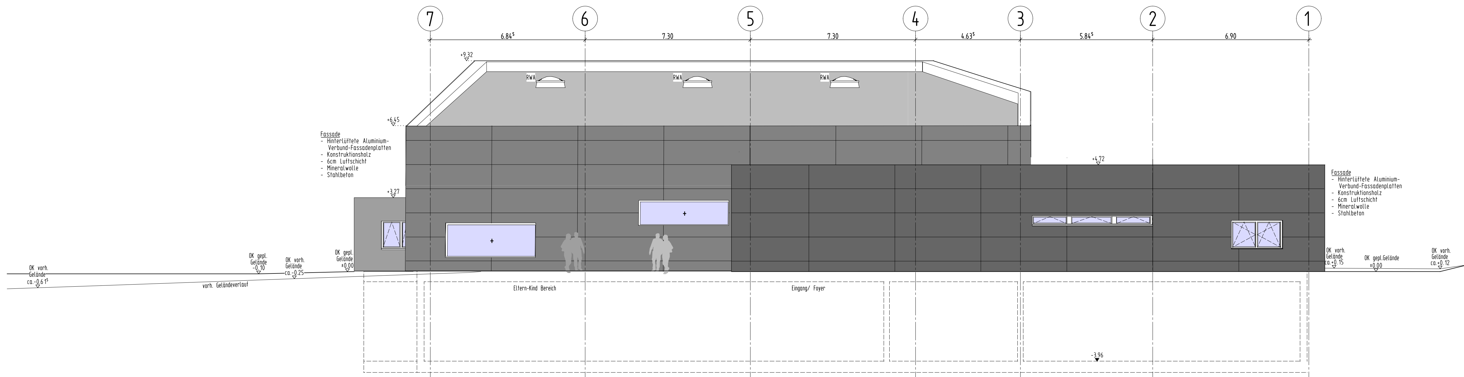
Ansicht Süd
